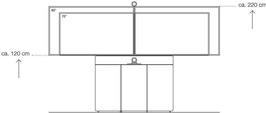
Wandmontiert
