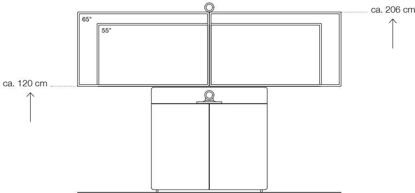
Wandmontiert
