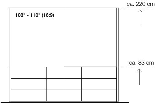
wandmontiert, dreitürig
