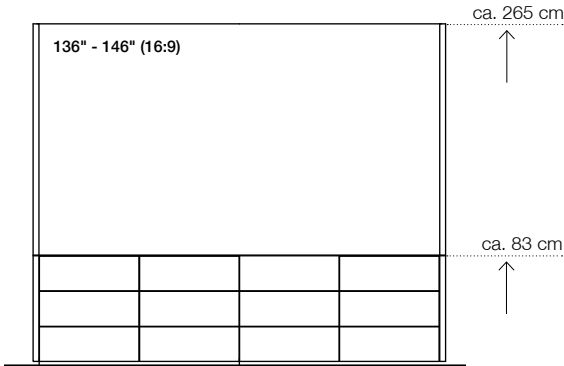
wandmontiert, viertürig
