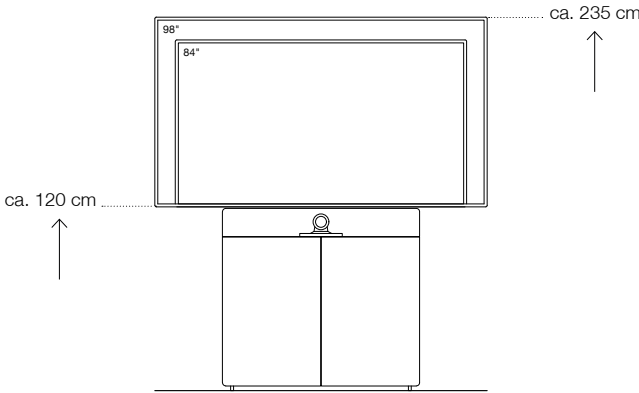
Wandmontiert
