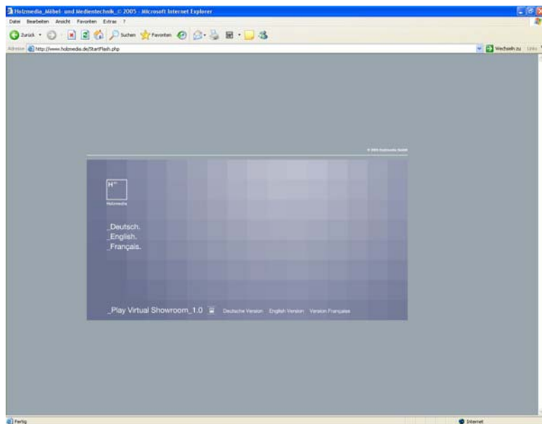
Bild 04: Startansicht
