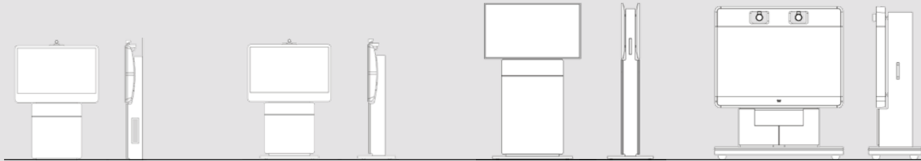
4 Stück Individuelle Medienstelen für Cisco MX200 mit 42"-Display, wandmontiert
