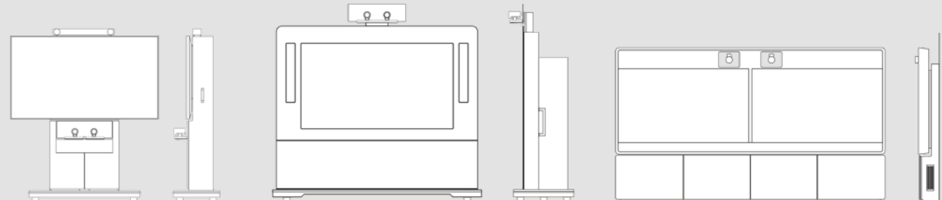
1 Stück Individuelle Medienstelen mit Cisco SX80, SpeakerTrack 60 und 95"-Display, mobil
